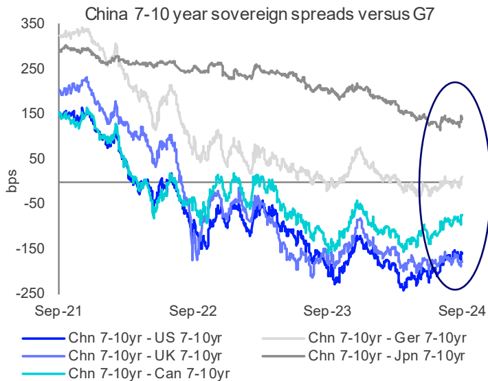
図 2: 中国の 7-10 年セクターの対 G7 スプレッド
